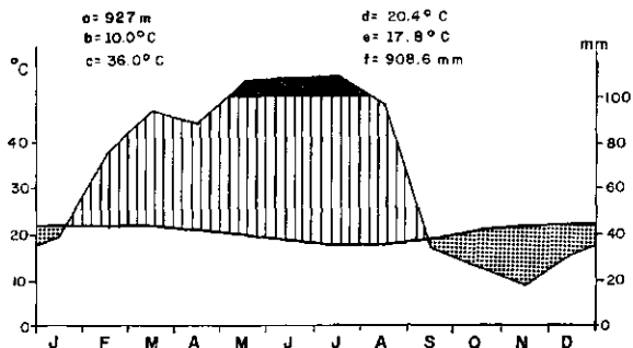
Fig.18.13- GARANHUNS (PE)- Clima SUB-QUENTE e SEMI-ÚMIDO - Com 5 meses secos do Tipo Mediterraneo
