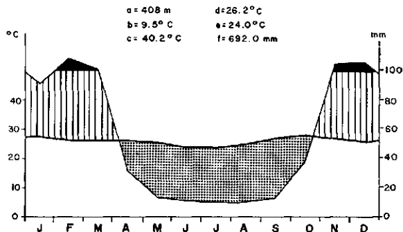
Fig.18.12-BARRA (BA)- Clima QUENTE e SEMI-ÁRIDO Com 7 meses secos do Tipo Tropical do Brasil Central
