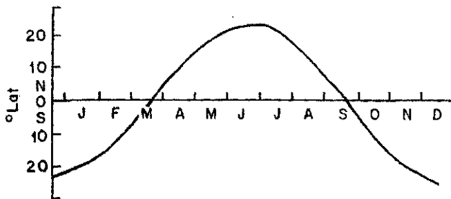
FIG. 2 — MARCHA ANUAL DA ALTURA ZENITAL DO SOL
