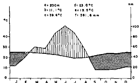
Fig. 18-7- TERESINA - (PI) - Clima QUENTE e SEMI-ÁRIDO Com 6 meses Sêcos - do Tipo Tropical da Zona Equatorial
