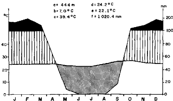
Fig.18.11-BARREIRAS (BA)- Clima QUENTE e SEMI-ÚMIDO Com 5 meses secos do Tipo Tropical do Brasil Central
