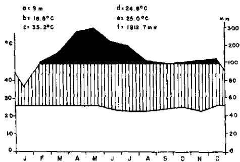
Fig. 18-4- SERTÃOZINHO - (AL) - Clima SEMI-ÁRIDO Com 6 meses Sêcos - do Tipo Mediterrâneo
