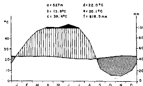
Fig. 18-6- BARRA DO CORDA - (MA) - Clima QUENTE e SEMI-ÚMIDO - Com 5 meses Sêcos - do Tipo Tropical da Zona Equatorial
