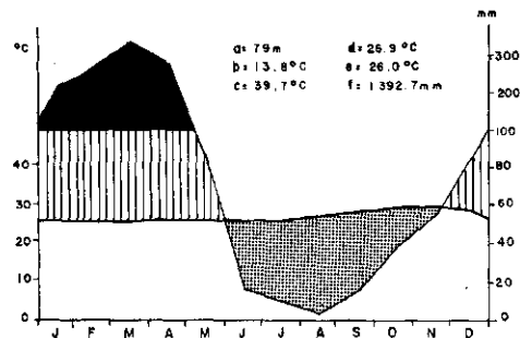
Fig. 18-7- TERESINA - (PI) - Clima QUENTE e SEMI-ÁRIDO Com 6 meses Sêcos - do Tipo Tropical da Zona Equatorial
