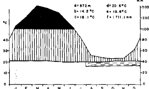
Fig. 18-8- QUIXERAMOBIM - (CE) - Clima QUENTE e SEMI-ÁRIDO - Com 7 meses Sêcos - do Tipo Tropical da Zona Equatorial
