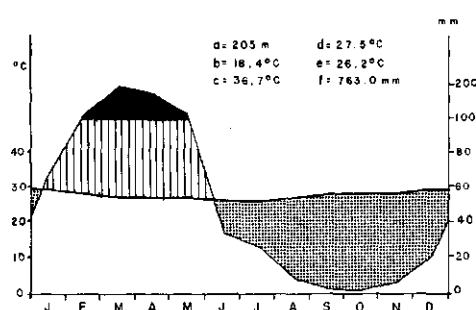
Fig. 18-8- QUIXERAMOBIM - (CE) - Clima QUENTE e SEMI-ÁRIDO - Com 7 meses Sêcos - do Tipo Tropical da Zona Equatorial
