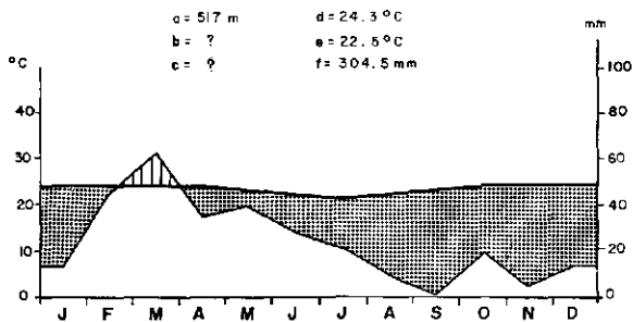
Fig.18.9 - SOLEDADE (PB)- Clima QUENTE e SEMI-ÁRIDO (Sub-desértico) Com 11 meses secos do Tipo Tropical da Zona Equatorial
