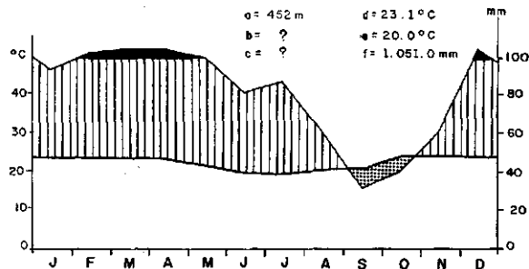
Fig.18.10- JACOBINA (BA)- Clima QUENTE e ÚMIDO Com 2 meses secos do Tipo Tropical do Brasil Central
