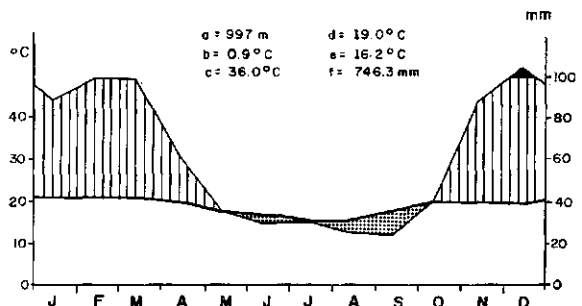
Fig.18.14- MORRO DO CHAPÉU (BA)- Clima SUB-QUENTE e SEMI-ÚMIDO - Com 5 meses secos do Tipo Tropical do Brasil Central
