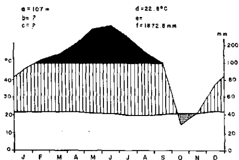
Fig. 18-5- GUARAMIRANGA - (CE) - Clima QUENTE e SUPER-ÚMIDO com Subseco - do Tipo Tropical da Zona Equatorial
