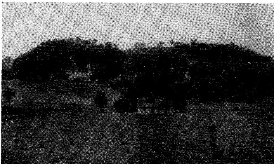
Foto 2 — "Verruga" calcária rochosa, 3 km ao norte de Matozinhos Colina calcária rochosa abrupta, surgindo de maneira insólita das ondulações suaves da região O alinhamento da escarpa corresponde provavelmente a uma falha, pondo em contato o calcário e as formações metamórficas A parte superior da parede calcária em saliência demonstra que a erosão é mais ativa na base que no alto
