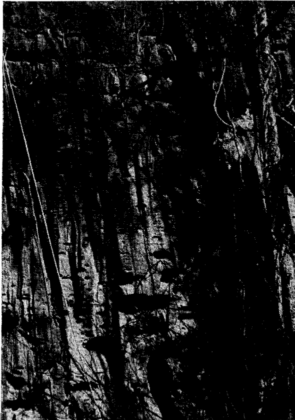
Foto 8 — Parede rochosa com caneluras, Nova Granja (M G) Combinação de caneluras e de alvéolos, na parte inferior do clichê (bancos de rochas compactas), e de caneluras e "lapiez" de juntas, na parte superior
