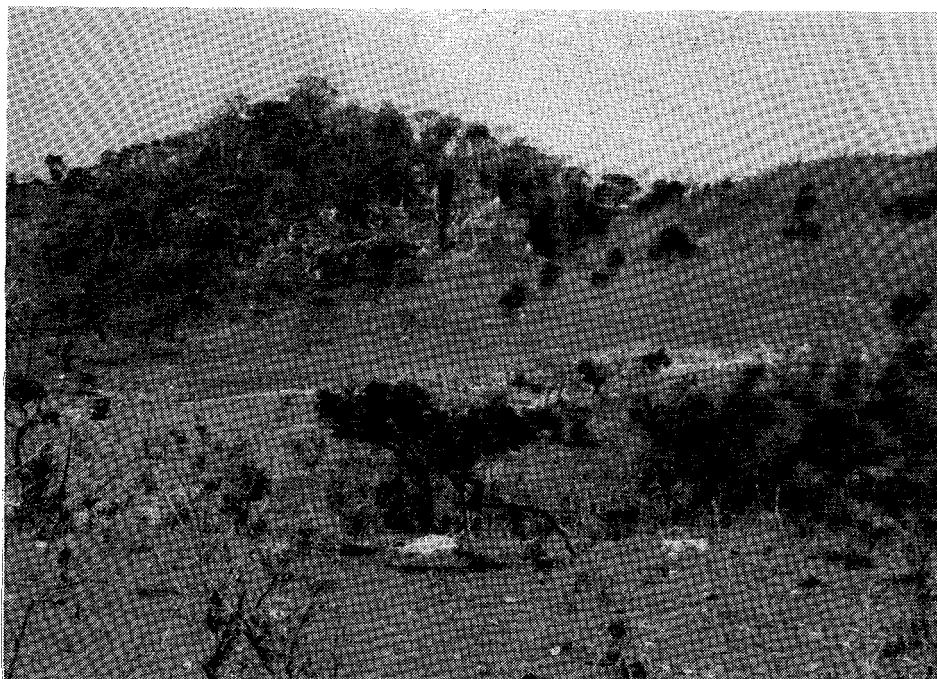
Foto 3 — Colina ruiforme calcária, em Sete Lagoas (M G) No primeiro plano e à direita, formas côncavo-convexas de colinas metamórficas com espessos solos de alteração No fundo, destacado pela erosão diferencial, um maciço calcário. Notar a cobertura florestal.
