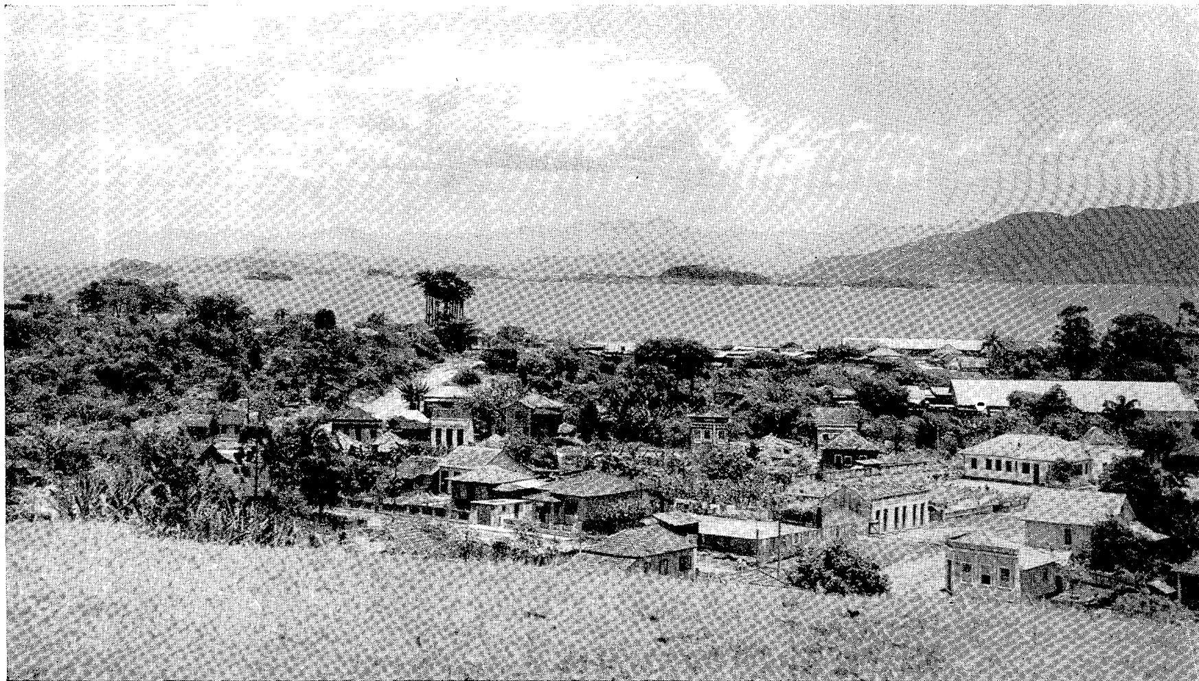
Fig. 3 — Perfil longitudinal do alinhamento de terraços constantes de pequenas ilhas dissecadas pela erosão marinha (wave cut terrace) Ao fundo, a serra do Mar (jalhada) A direita plataforma de erosão subaérea que entesta a península do Sai. A esquerda trecho da parte sul da cidade de São Francisco do Sul.
