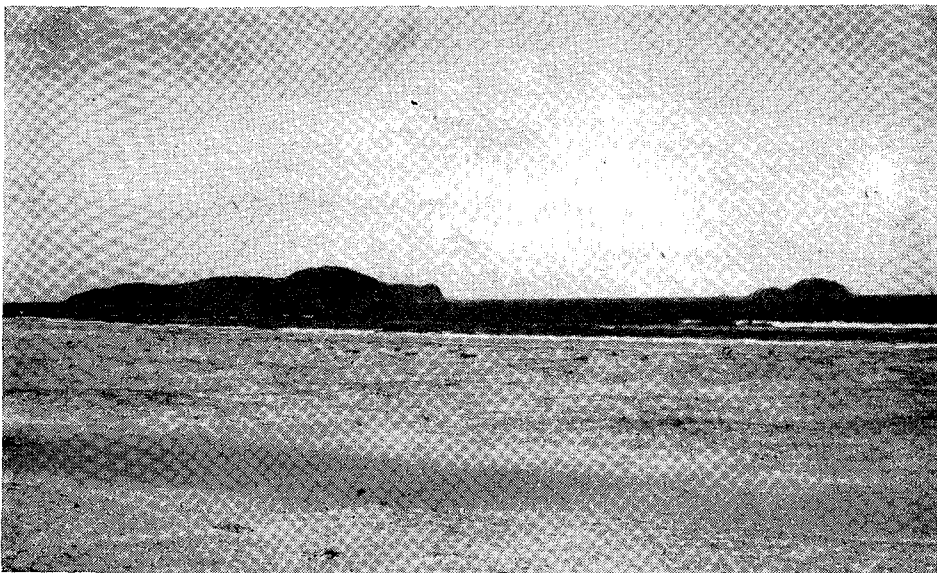
Fig 8 — Grupo das ilhas Remédios. Constitui a parte emergida mais avançada de uma plataforma submersa. Observe-se o contorno terraceado das ilhas, que formaria mais um nível costeiro da ordem de 30-60 metros, correspondente a outros da mesma ordem, situados na ilha de São Francisco
