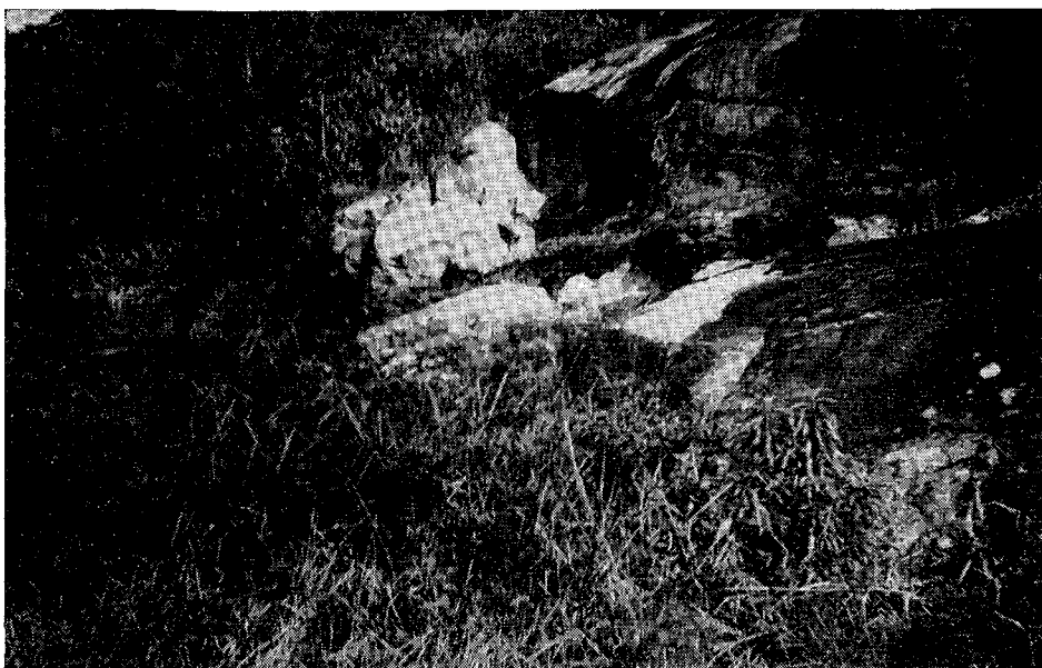
Fig 4 — Afloramento de biotita-hornblenda-gnaiss, no morro do Rocio Observe-se diaclasamento do bloco Orientação N 45 NE (Foto do autor)
