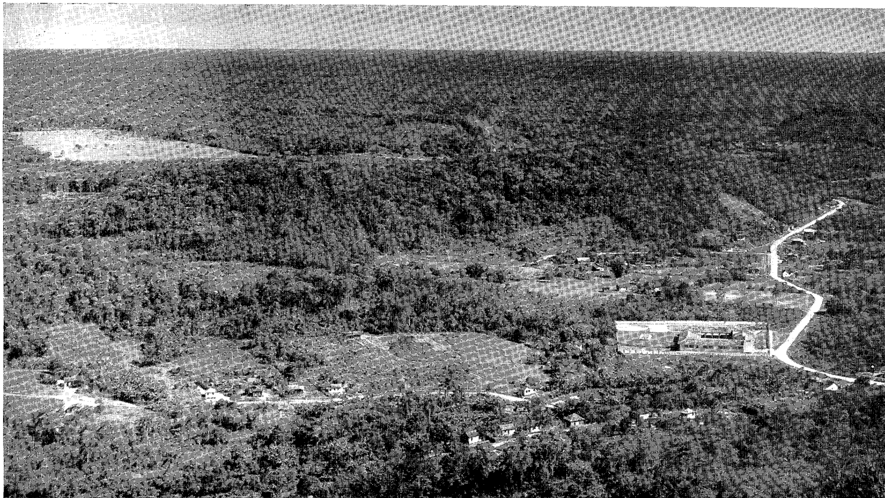
Fig. 11 — Panorama da parte oriental da ilha de São Francisco do Sul constituída de sedimentos arenosos construídos de antigas restingas formadas a custa do mar (wave built terrace) Ao fundo, o oceano Atlântico.
