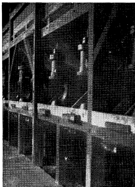
Fig. 16 — Parte das 40 máquinas de quebrar coquilhos, movidas a vapor, em abandono na fábrica de Queiru.
