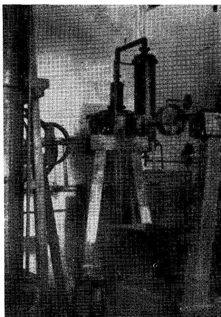
Fig. 17 — Caldeira para destilação da casca, alambique, colunas de destilação e um filtro-prensa de três placas. Tudo abandonado na fábrica de Queiru.
