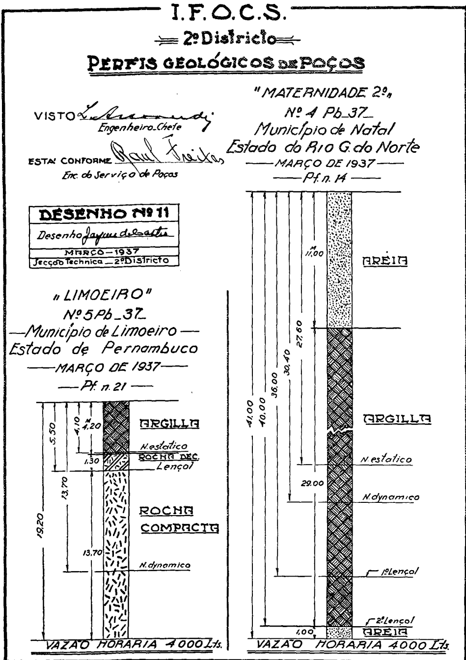
Fig. 17 — Perfil geológico de um poço aberto em Limoeiro
