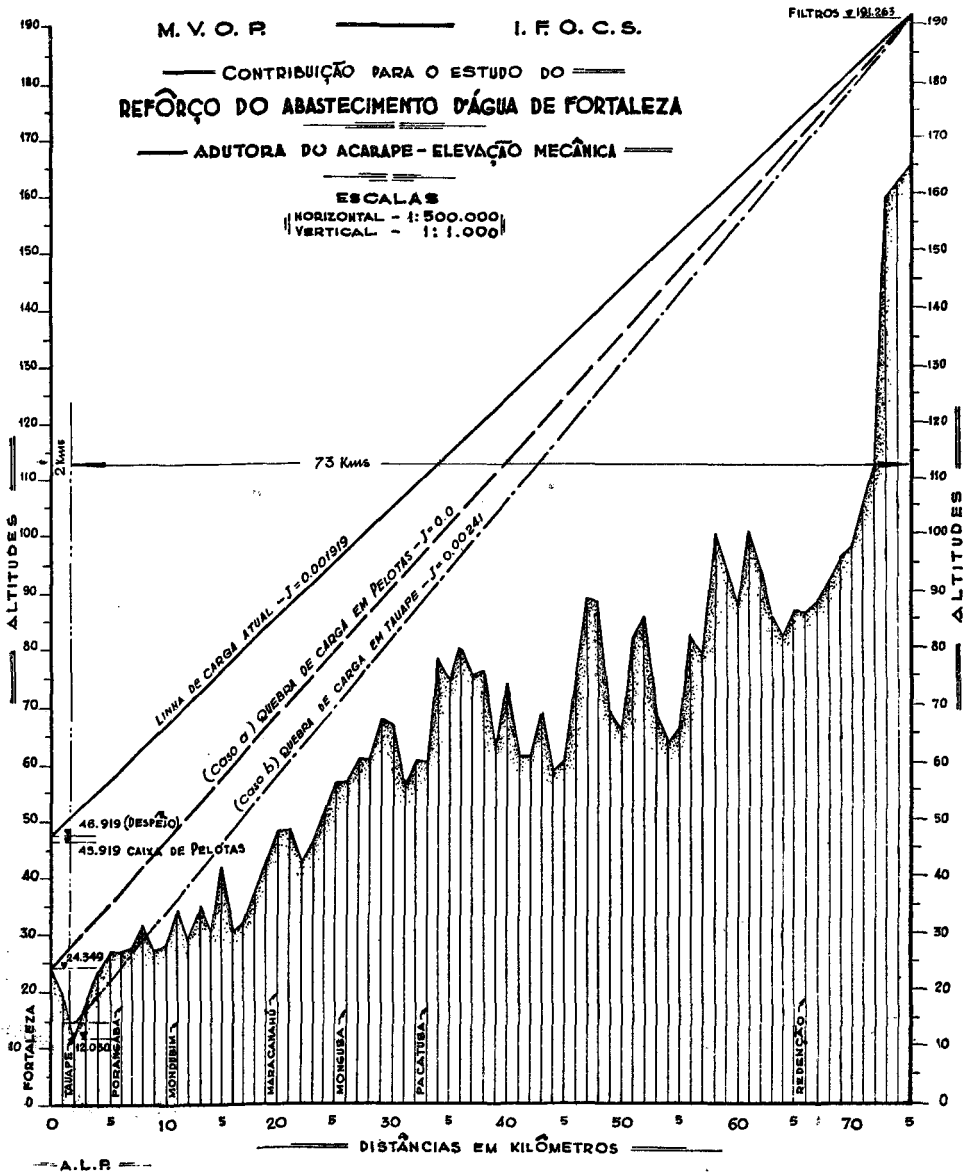
Fig. 12 — Adutora do Acarape
