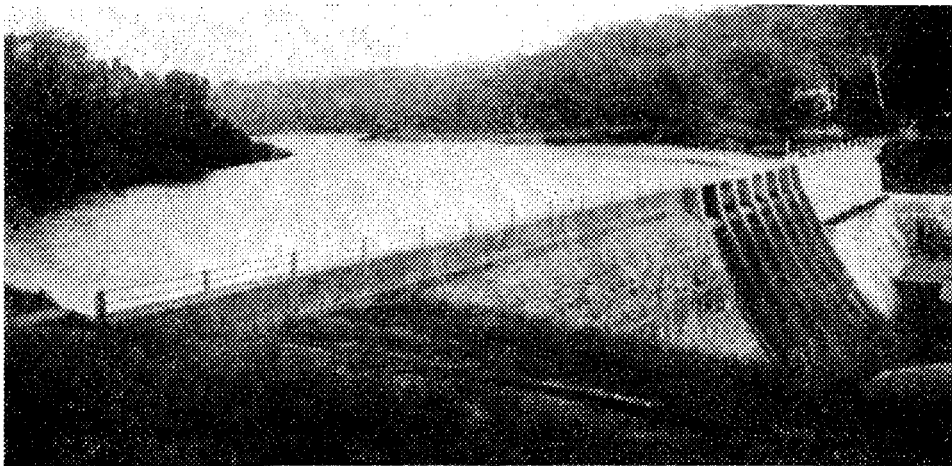
Fig. 2 — Barragem do rio Cobre com 141 metros de comprimento e 18 de altura. Armazena 2.340.000 metros cúbicos d'água
