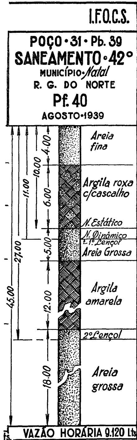
Fig. 6 — Poço perfurado em Natal Perfil geológico
