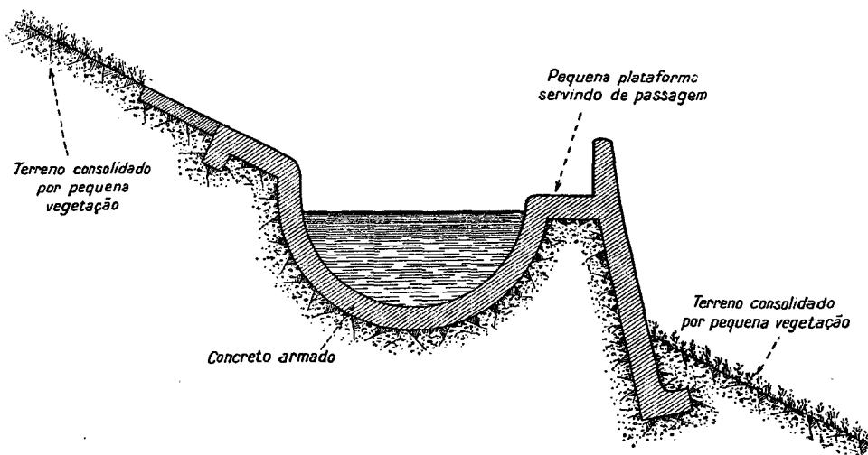
Fig. 21 — Perfil mostrando a localização das barragens e reservatórios
