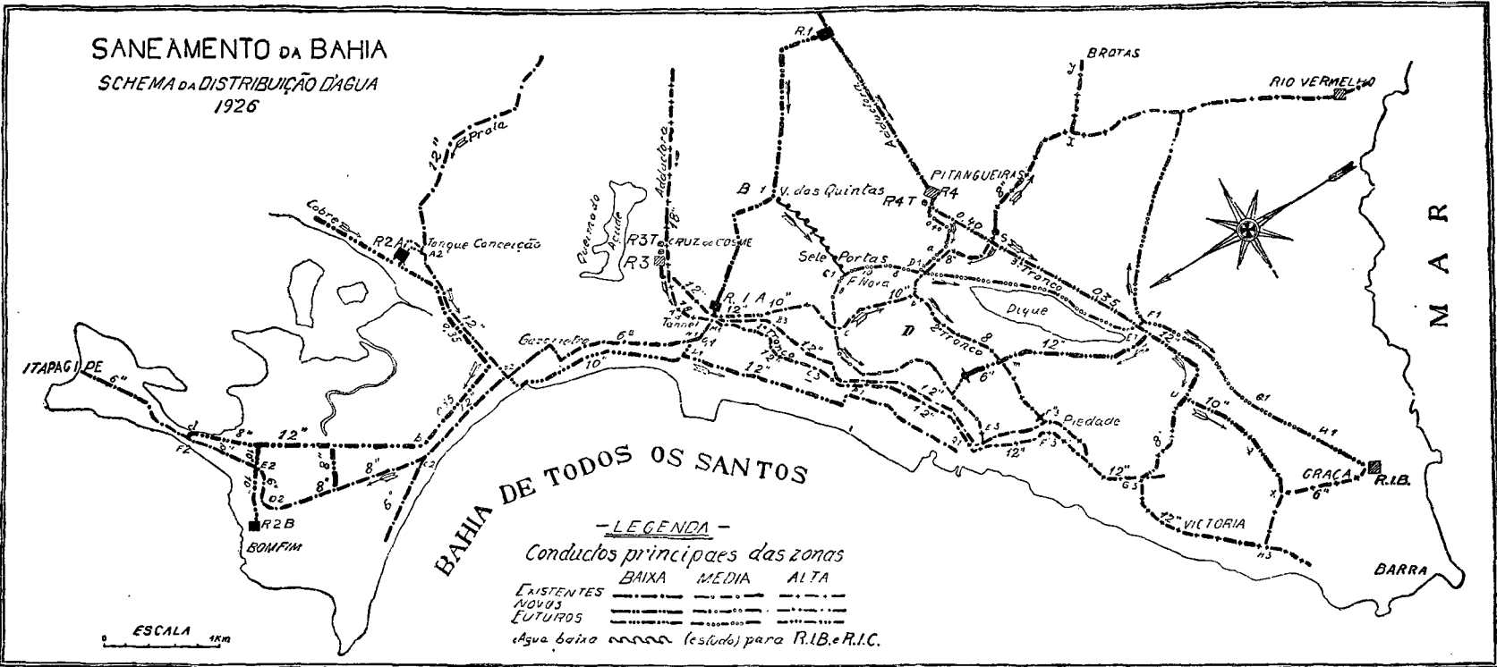
Fig. 4 — Posição dos reservatórios
