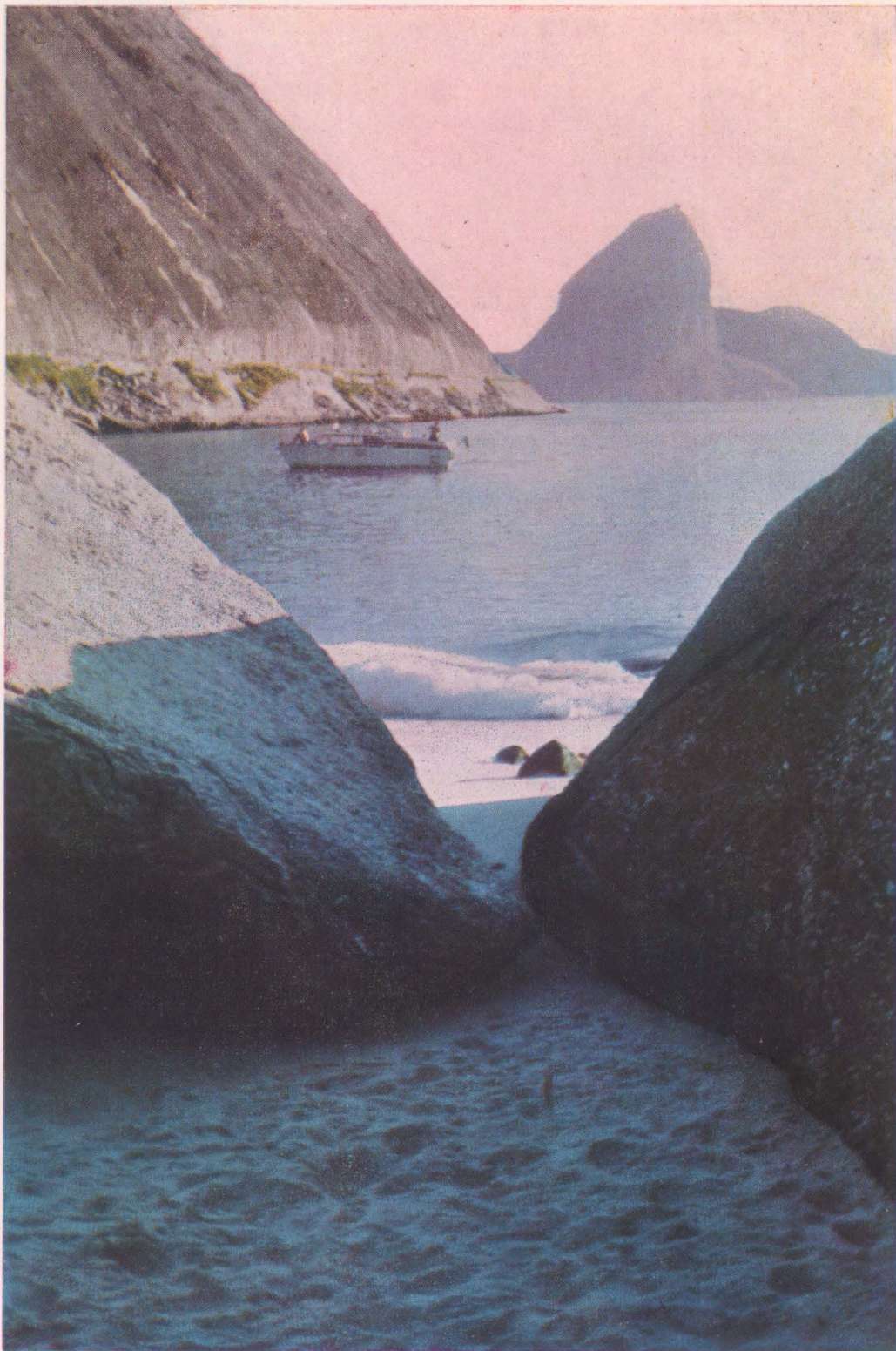
PONTOES GNAISSICOS DO CONTORNO DA GUANABARA
