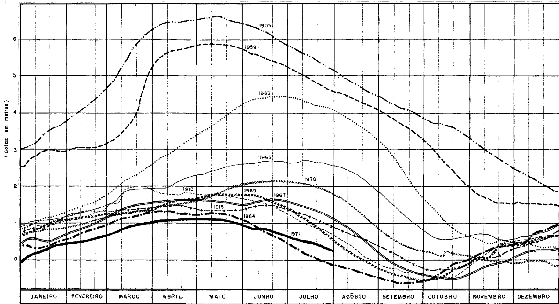
RIO PARAGUAI EM LADÁRIO FLUVIOGRAMA DE COTAS MÉDIAS DIÁRIAS
